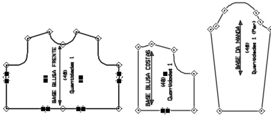
Figura 5: Moldes da blusa Fonte: Elaborado pelas autoras (2021)
