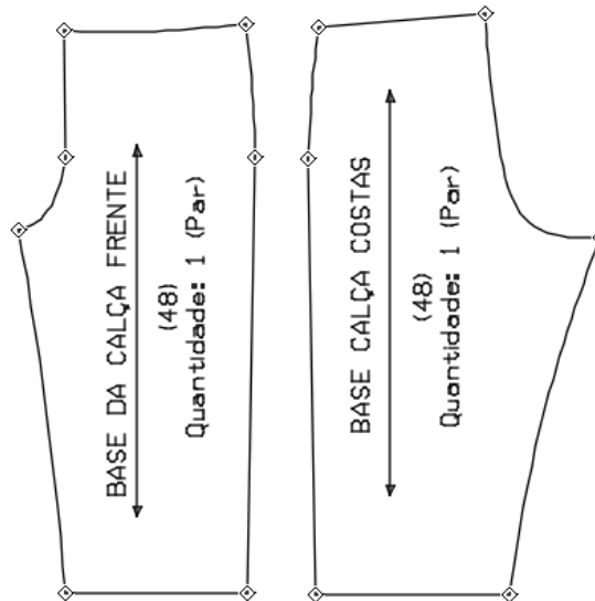
Figura 6: Moldes da calça Fonte: Elaborado pelas autoras (2021)
